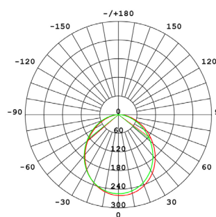
CURVA FOTOMETRICA
